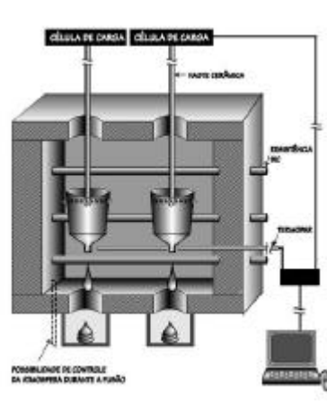
Figura 7 Diagrama esquemático do equipamento para avaliação da taxa de fusão
