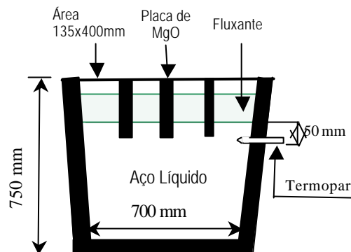
Figura 3 – Diagrama esquemático do equipamento utilizado. (Adaptado da ref. 5)
