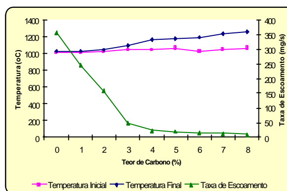
Figura 9. Gráfico demonstrando os resultados obtidos com (a) adição de carbono através do Negro de Fumo e (b) através do Coque na avaliação da velocidade de fusão.
